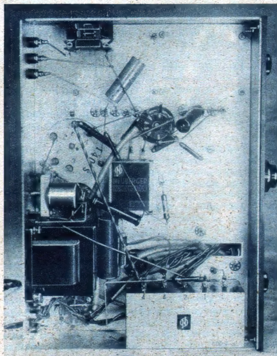
Die Unterficht des Gigannt gekennzeichnet durch ihre überfichtliche Leitungsführung. (Aufnahme Wacker)
