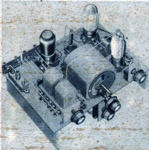
Der englische Bastler ist sehr konservativ. Er baut noch auf Sperrholz, nimmt Aufbausockel und führt auch die Verdrahtung oberhalb des Chassis aus. Zu beachten auch die Schraubklemmen zum Anschluß der Stromquellen statt der bei uns üblichen Buchfen. (Werkphoto Graham Farish Ltd.)
