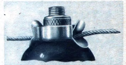
Antennenlitzen aus Aluminium verlangen besonders konstruierte Armaturen. (Werkphoto Wiff)
